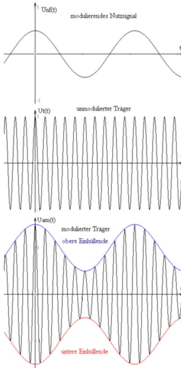
Abbildung 1 Quelle: http://de.wikipedia.org/wiki/Bild:Amplitudenmodulation3.png
